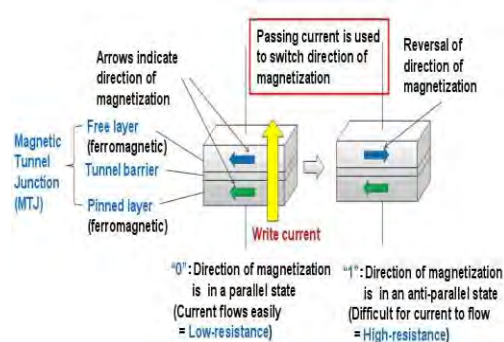
2. 自旋磁矩
