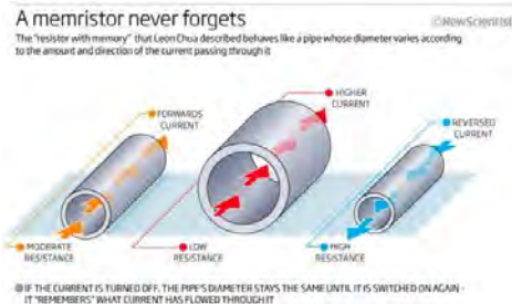
4. 忆阻器
