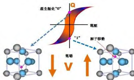
3. 铁电材质
