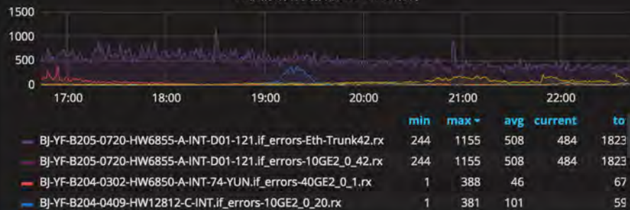
YF机房所有交换机 IN Error统计
