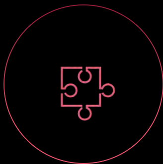
数据应用
