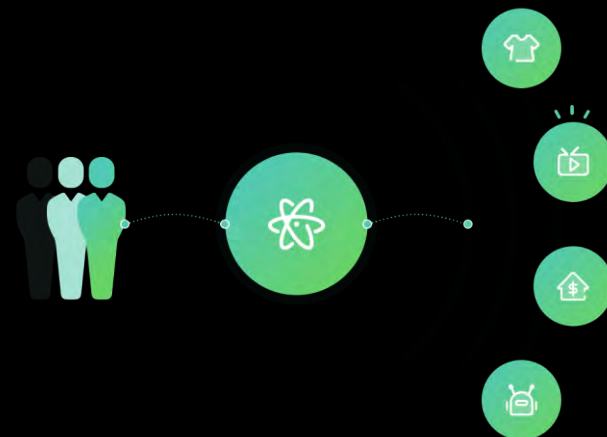
推荐引擎
