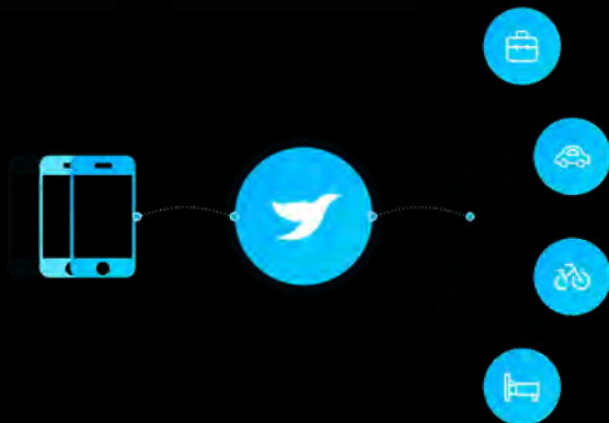
Myna
