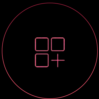
数据服务
