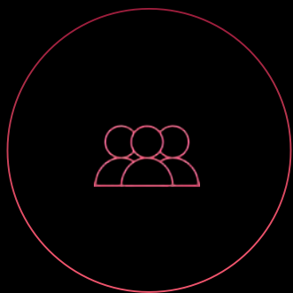
人群数据
