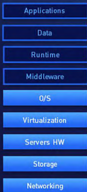
IaaS
