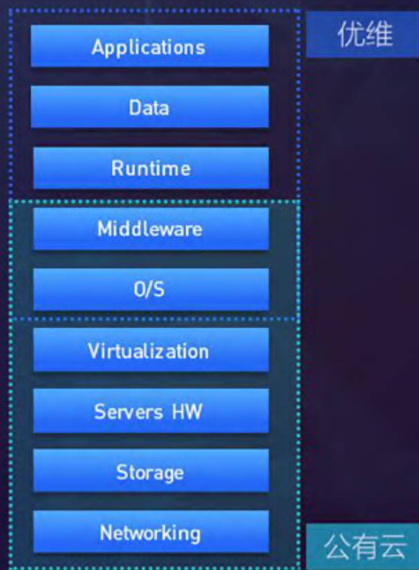
SaaS
