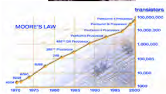
摩尔定律
