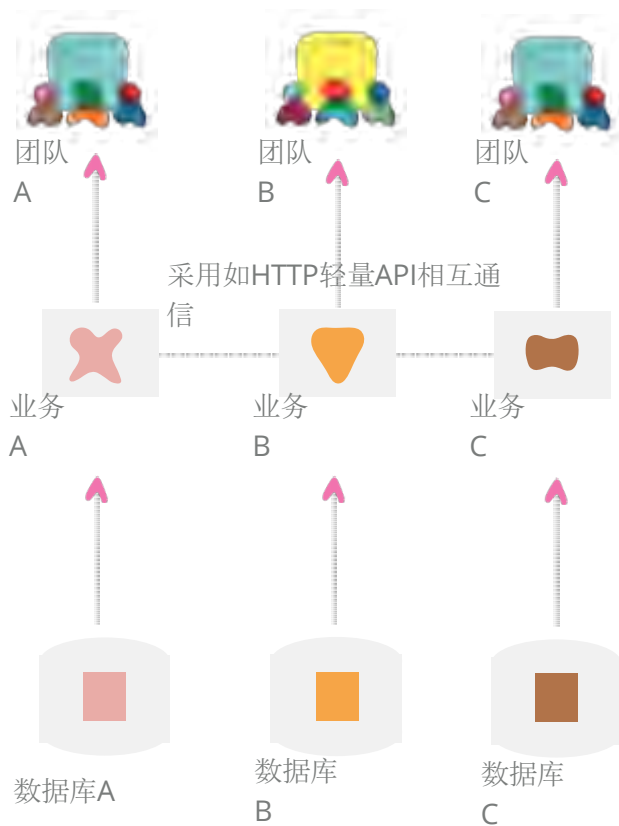
微服务架构
