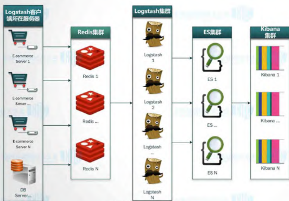
ELK服务部署拓扑图
