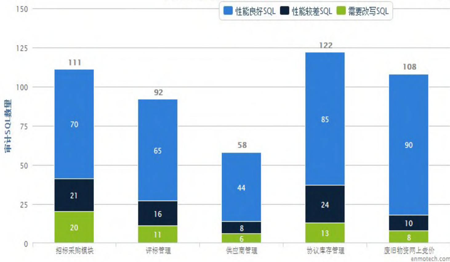
2012-11~2013-04审计SQL
