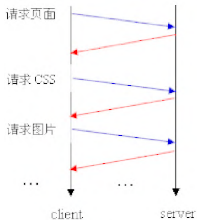
HTTP实现
