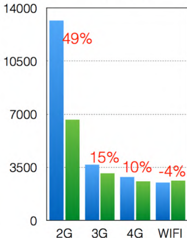
连接复用
