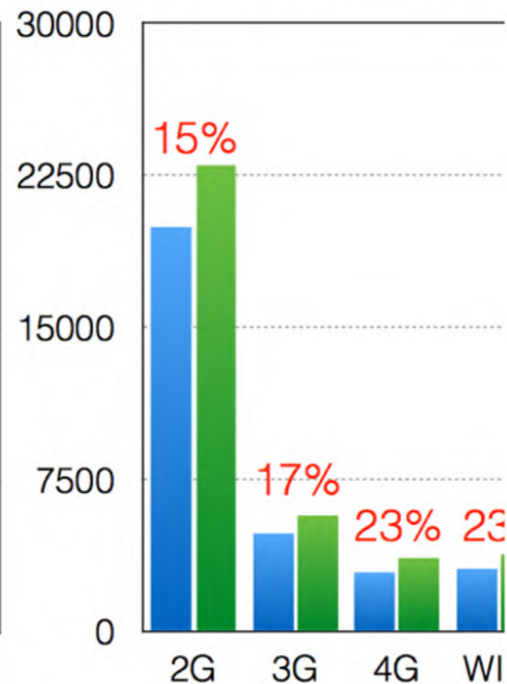
连接不复用
